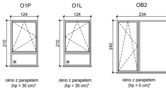
Schemat okien w widoku od zewnątrz:
