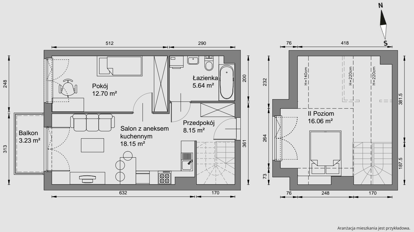
RZUT KONDYGNACJI
