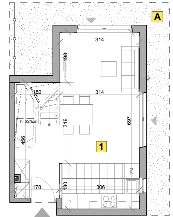
RZUT PARTERU
