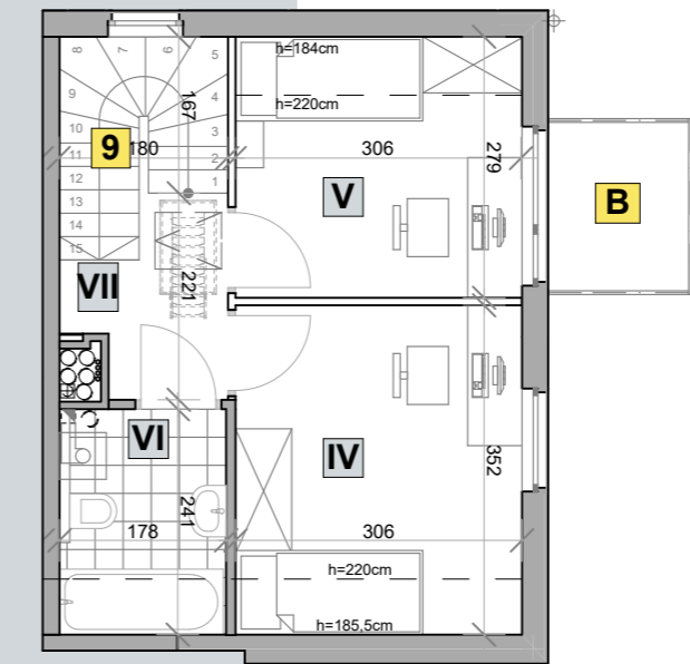
RZUT PIĘTRA +2 - aranżacja opcjonalna
