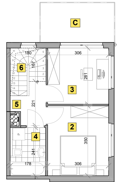
RZUT PIĘTRA +1
