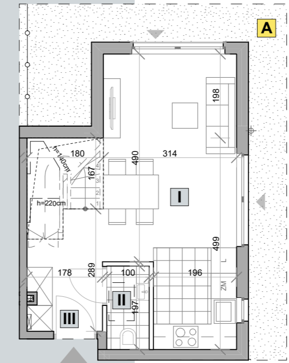
RZUT PARTERU - aranżacja opcjonalna
