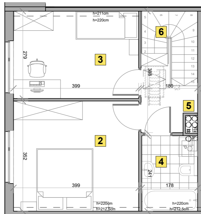
RZUT PIĘTRA +1
