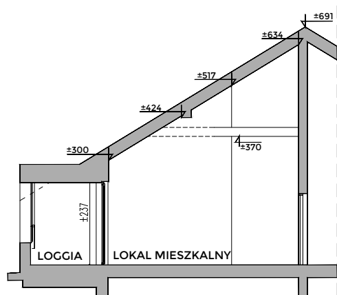
PRZEKRÓJ A-A
