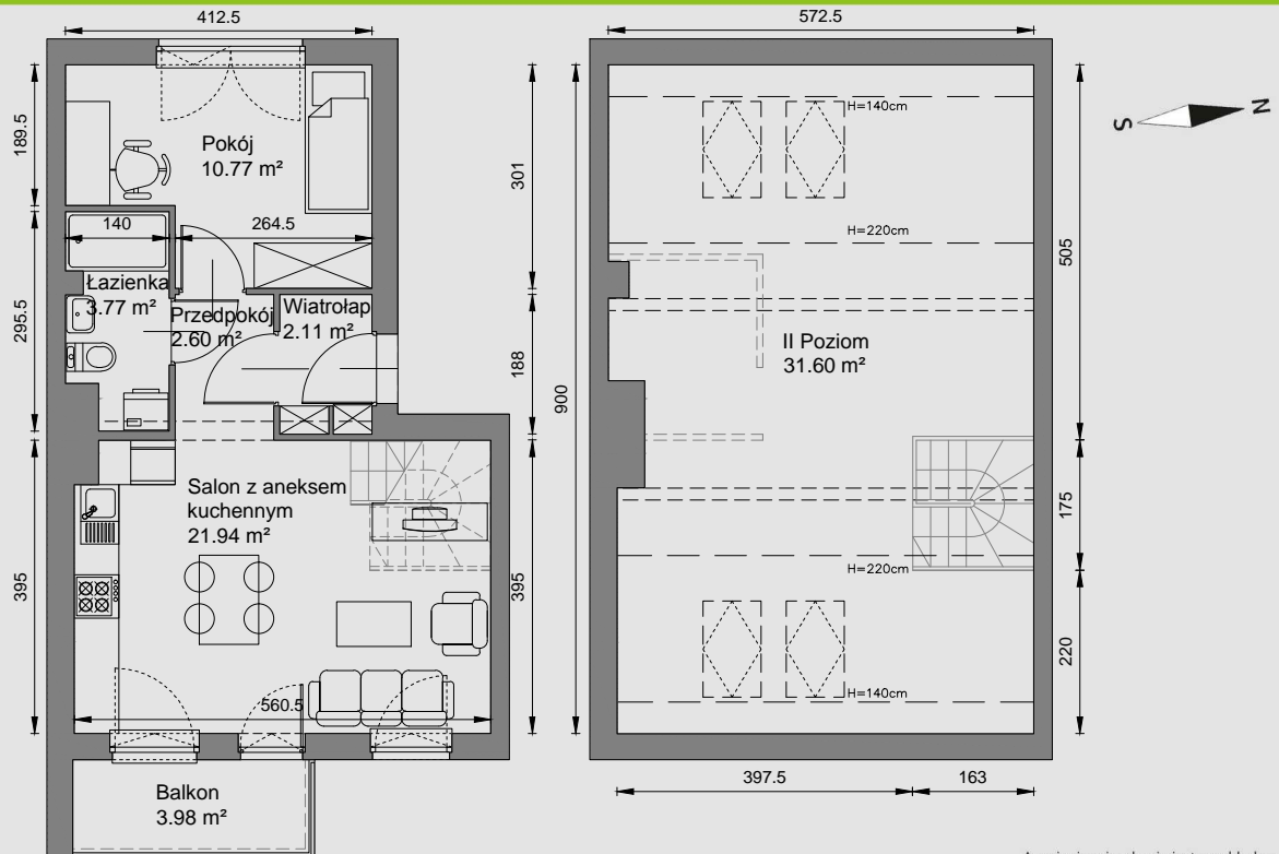
RZUT KONDYGNACJI
