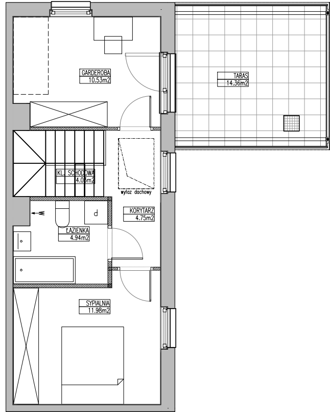
PIĘTRO
