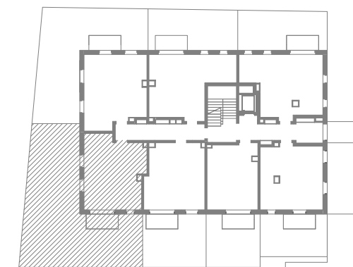
rzut kondygnacji z zaznaczeniem Apartamentu oraz jego położeniem
