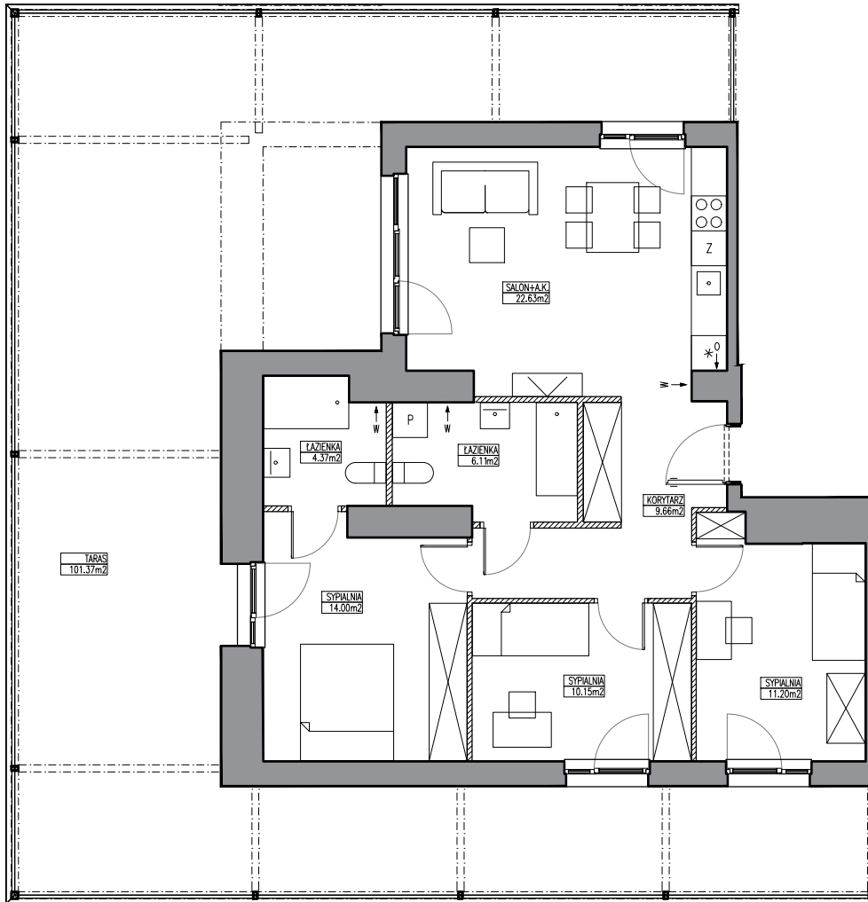
SCHEMAT LOKALU MIESZKALNEGO NA PIĘTRZE
