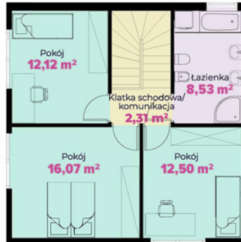
PIĘTRO
