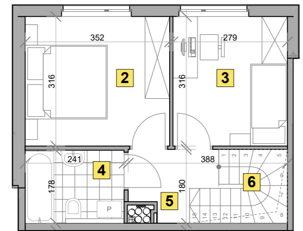
RZUT PIĘTRA +1
