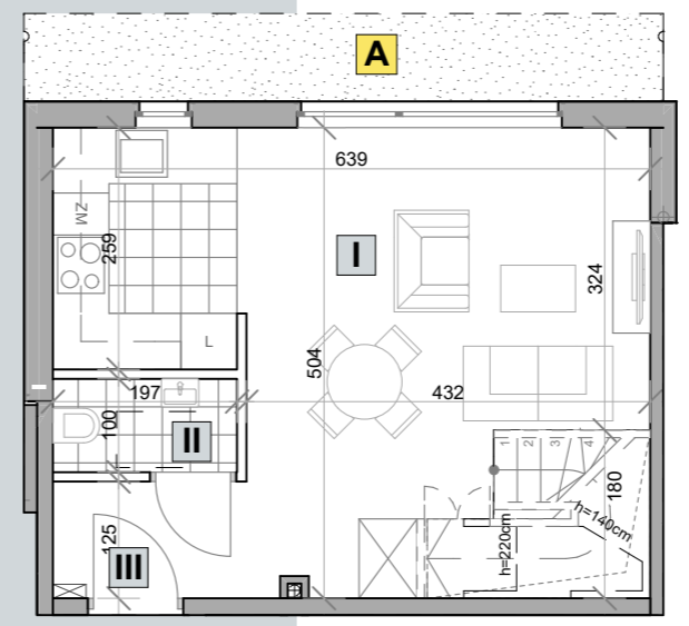
RZUT PARTERU - aranżacja opcjonalna
