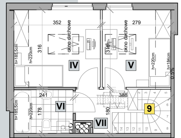
RZUT PIĘTRA +2 - aranżacja opcjonalna
