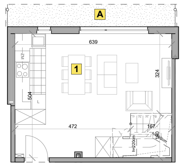
RZUT PARTERU - aranżacja podstawowa
