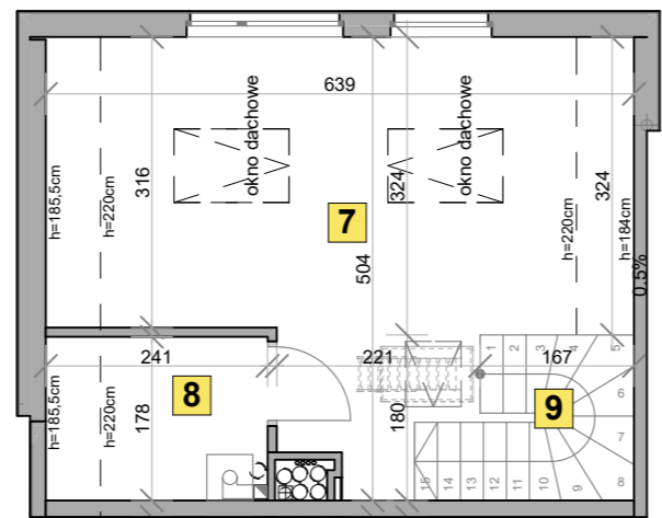
RZUT PIĘTRA +2 - aranżacja podstawowa
