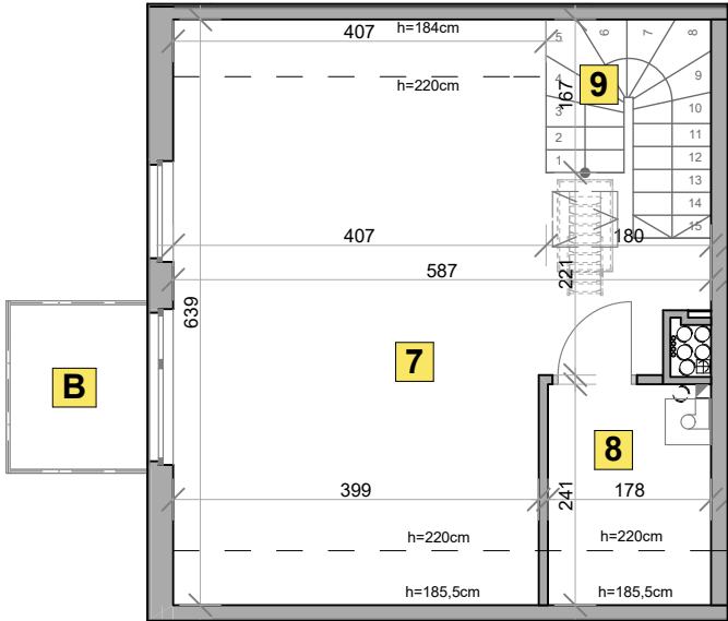
RZUT PIĘTRA +2 - aranżacja podstawowa
