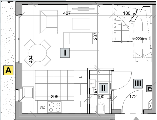
RZUT PARTERU - aranżacja opcjonalna
