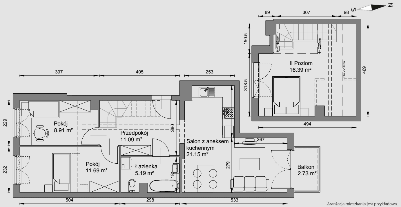
RZUT KONDYGNACJI
