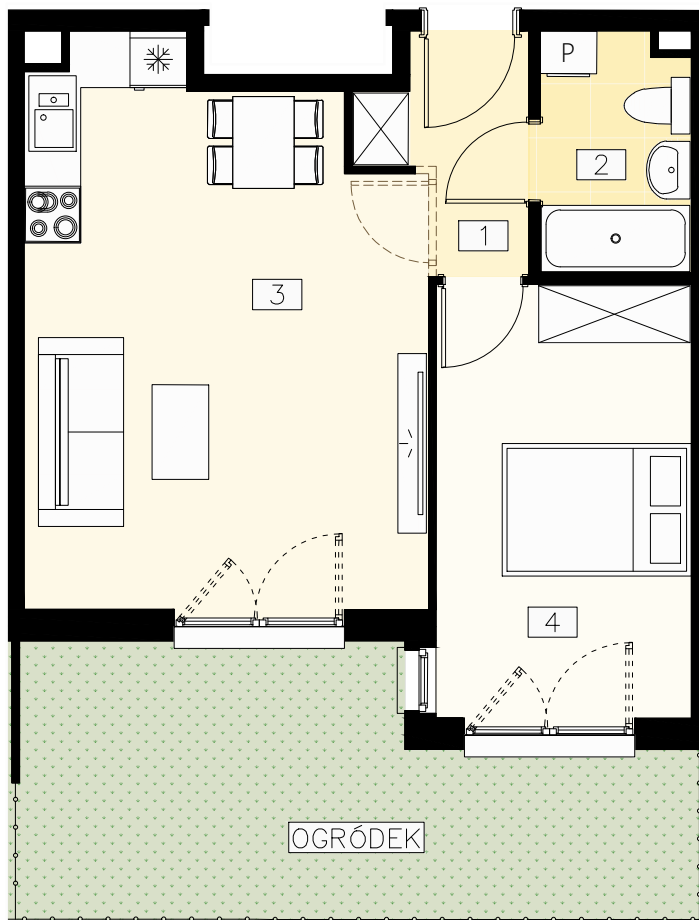
RZUT KONDYGNACJI
