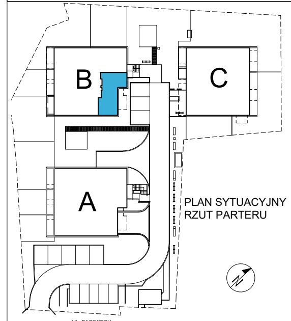
PLAN SYTUACYJNY RZUT PARTERU
