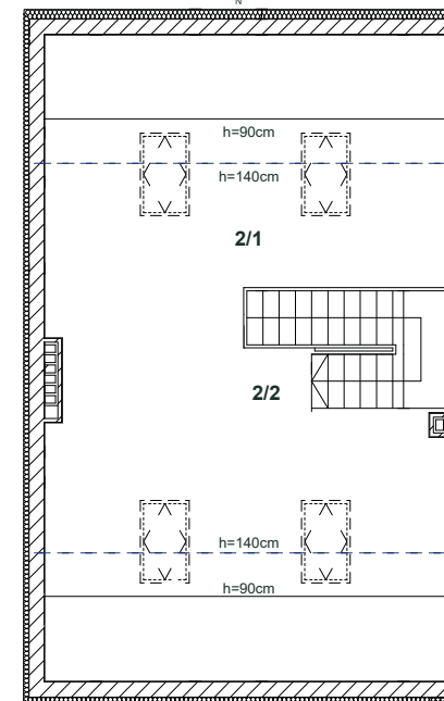
RZUT PODDASZE
