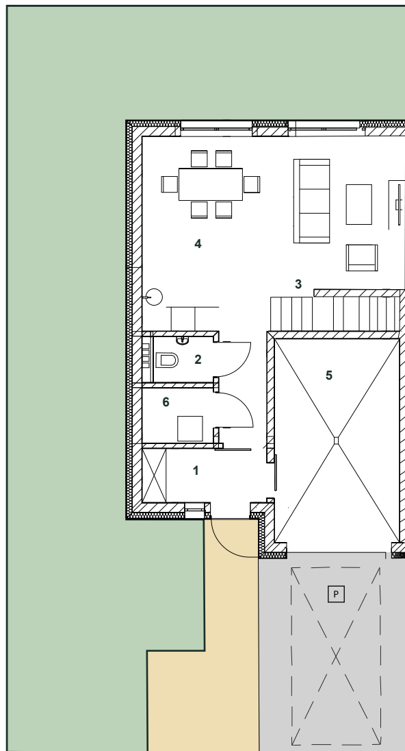
RZUT PARTER
