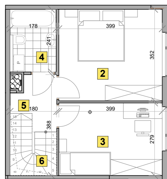
RZUT PIĘTRA +1
