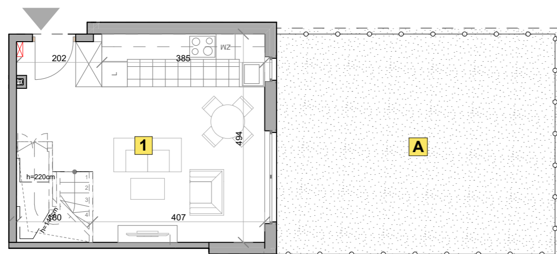
RZUT PARTERU - aranżacja podstawowa
