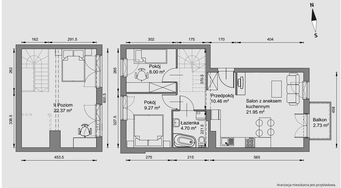
RZUT KONDYGNACJI
