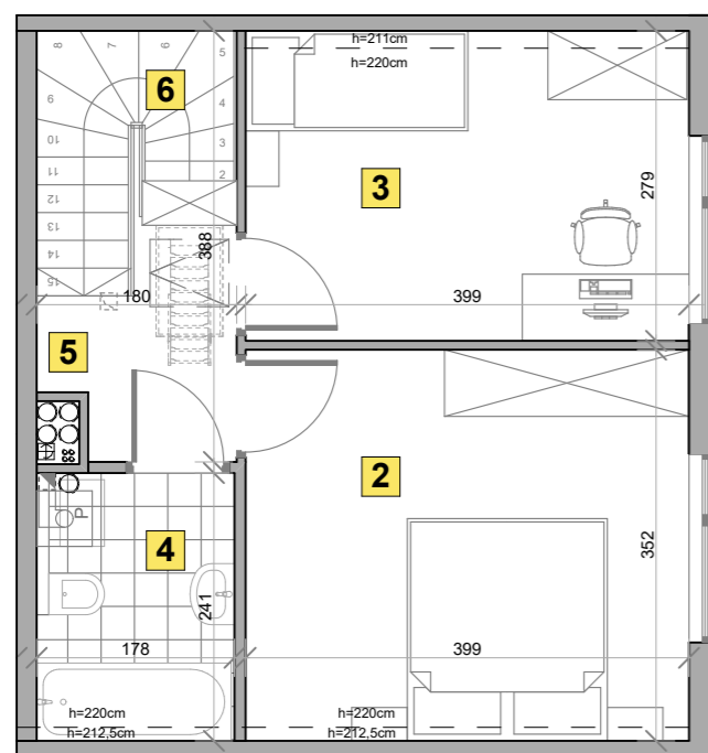
RZUT PIĘTRA +1
